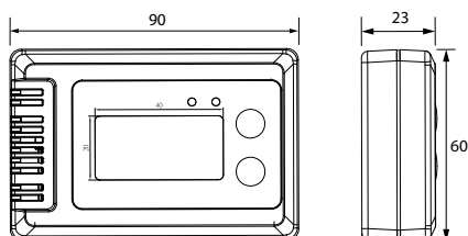
Typ TL-1D
